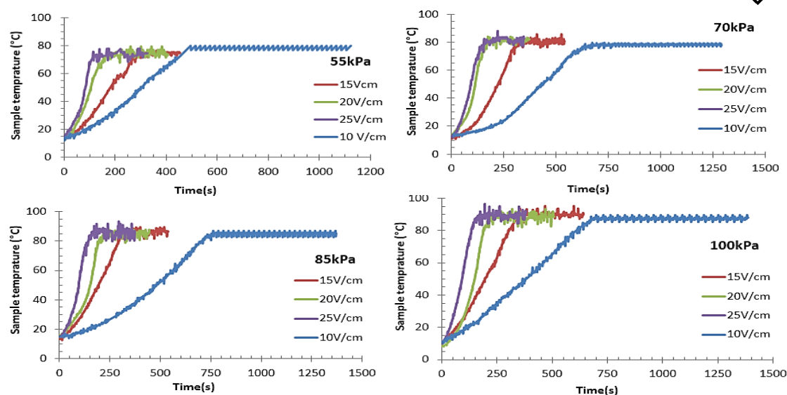
شکل ۳. تغییرات دمایی نمونه‌های تغلیظ‌شده شیر خرمای فرایند گرمایش
