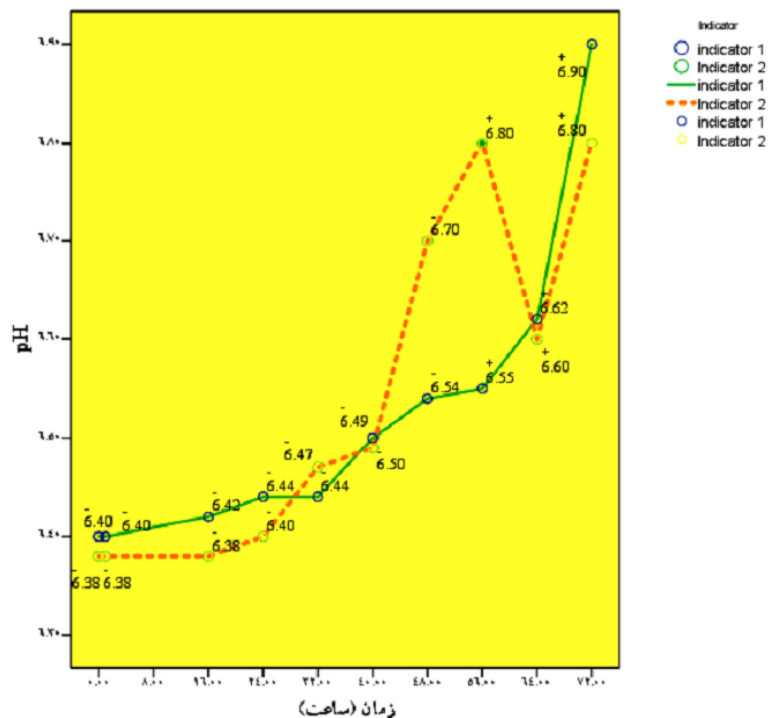
شکل (6) ارتباط pH و تغییر رنگ ایجادشده توسط معرف‌ها (3 mL) در گوشت مرغ بسته‌بندی شده در 4 \pm 2^\circ\text{C} : اندیکاتور 1: بروموکروزول گرین، اندیکاتور 2: فنل رد
