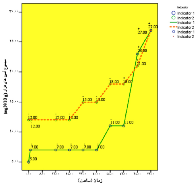
شکل (5) ارتباط مجموع آمین‌های فرار و تغییر رنگ ایجادشده توسط معرف‌ها (3 mL) در گوشت مرغ بسته‌بندی شده در 4 \pm 2^\circ\text{C} : اندیکاتور 1: بروموکروزول گرین، اندیکاتور 2: فنل رد
