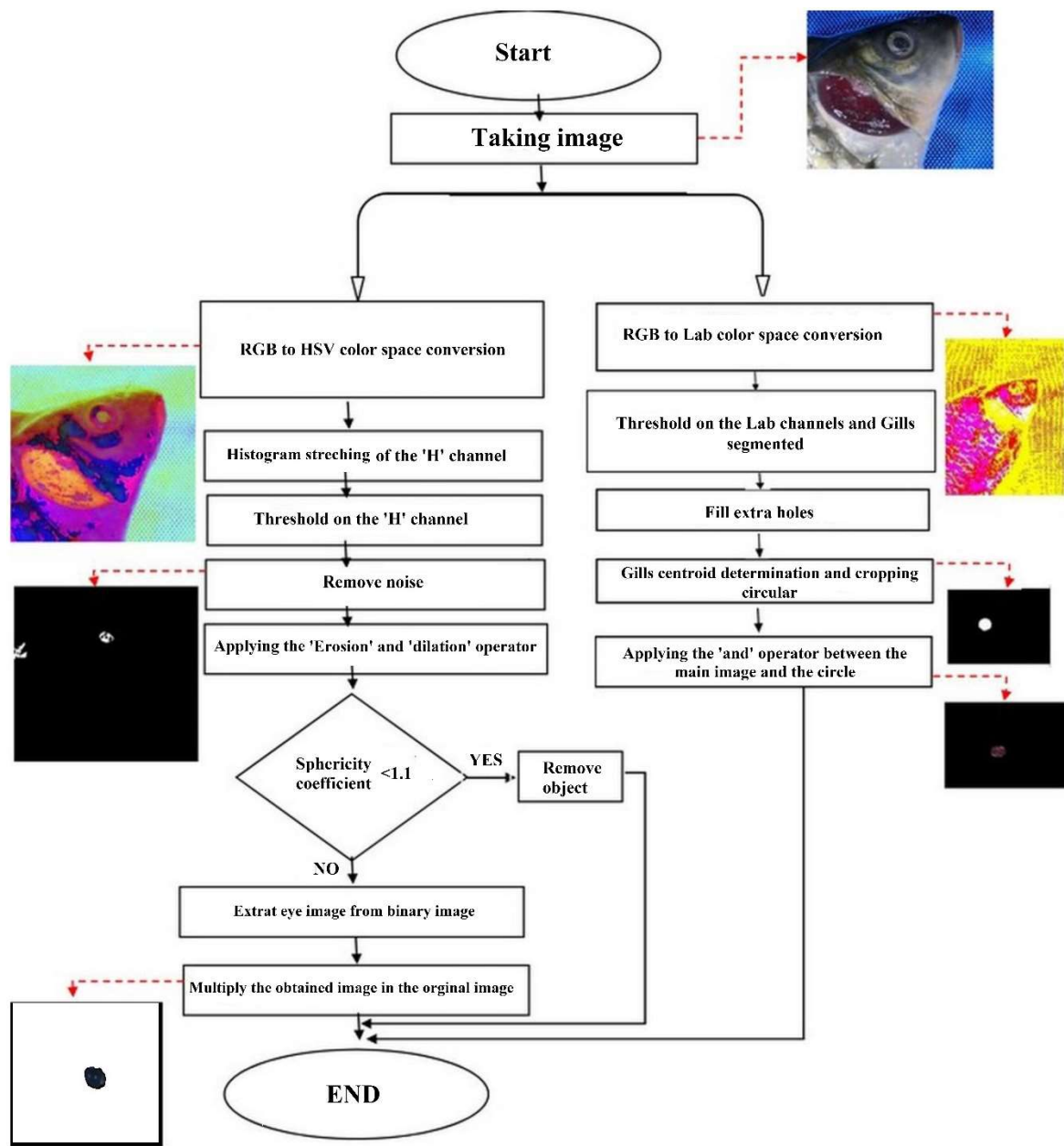
شکل (۱) فلوجارت روند پردازش تصویر
