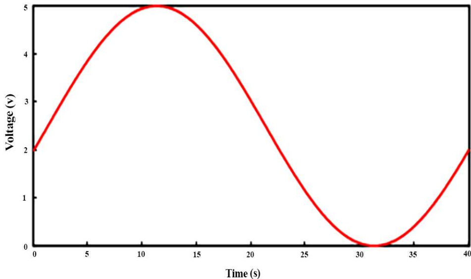
شکل (۱) الگوی ولتاژی اعمال شده به ریزگرمنک حسگرها تحت مدولاسیون دمایی
