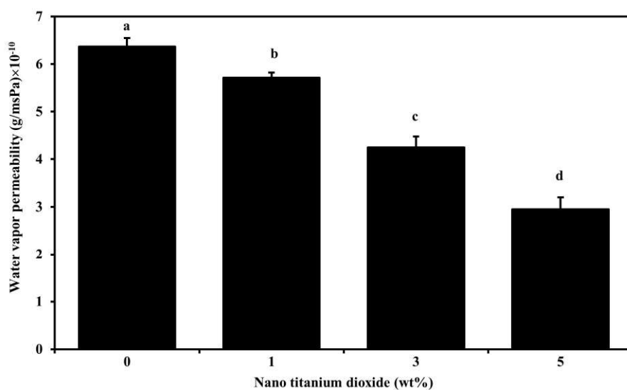
شکل (۶) میزان نفوذ پذیری به بخار آب فیلم‌های کاساوا و ژلاتین با غلظت‌های مختلف نانو دی اکسید تیتانیوم Fig. 6 Water vapor permeability of the cassava starch and bovine gelatin films with different nano titanium dioxide contents
