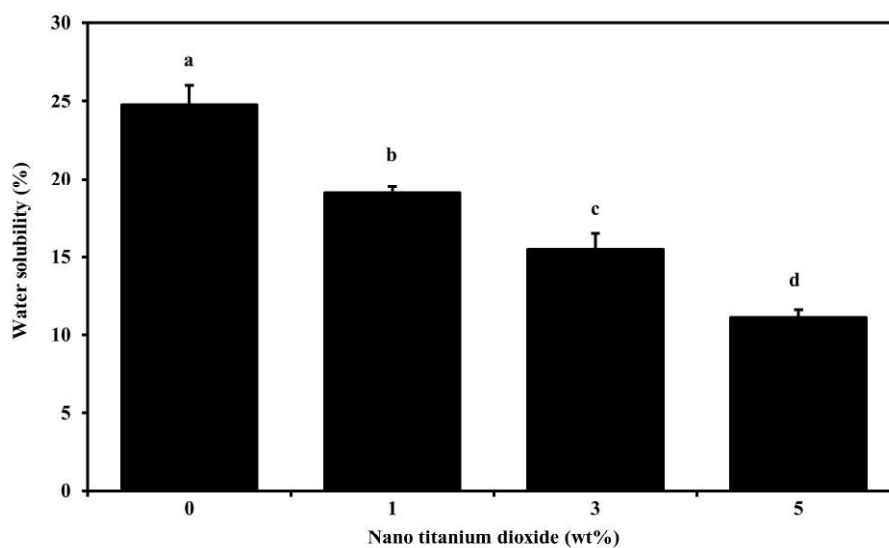
شکل (۵) میزان حلالیت در آب فیلم‌های نشاسته کاساوا و ژلاتین، با غلظت‌های مختلف نانو دی اکسید تیتانیوم Fig. 5 Water solubility of the cassava starch and bovine gelatin films with different nano titanium dioxide contents
