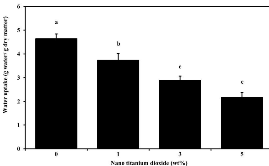
شکل (۴) میزان جذب آب فیلم‌های نشاسته کاساوا/ژلاتین، با غلظت‌های مختلف نانو دی اکسید تیتانیوم
