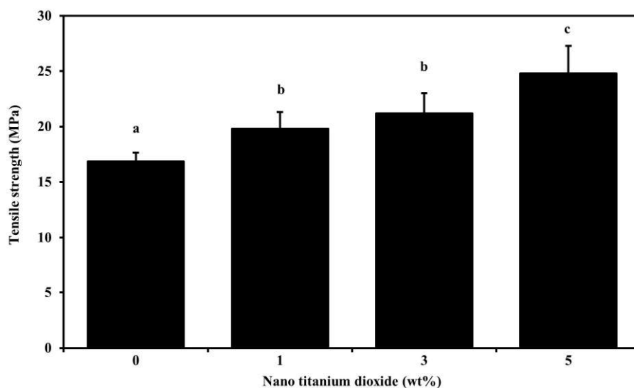
شکل (۱) نمودار مقاومت به کشش فیلم‌های نشاسته کاساوا و ژلاتین با غلظت‌های مختلف نانو دی اکسید تیتانیوم
