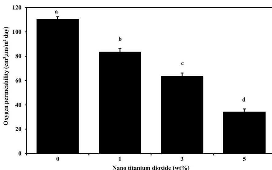
شکل (۷) میزان نفوذ پذیری به اکسیژن فیلم‌های کاساوا و ژلاتین با غلظت‌های مختلف نانو دی اکسید تیتانیوم
