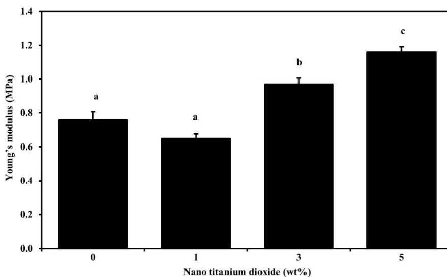
شکل (۳) نمودار مدول یانگ فیلم‌های نشاسته کاساوا و ژلاتین با غلظت‌های مختلف نانو دی اکسید تیتانیوم
