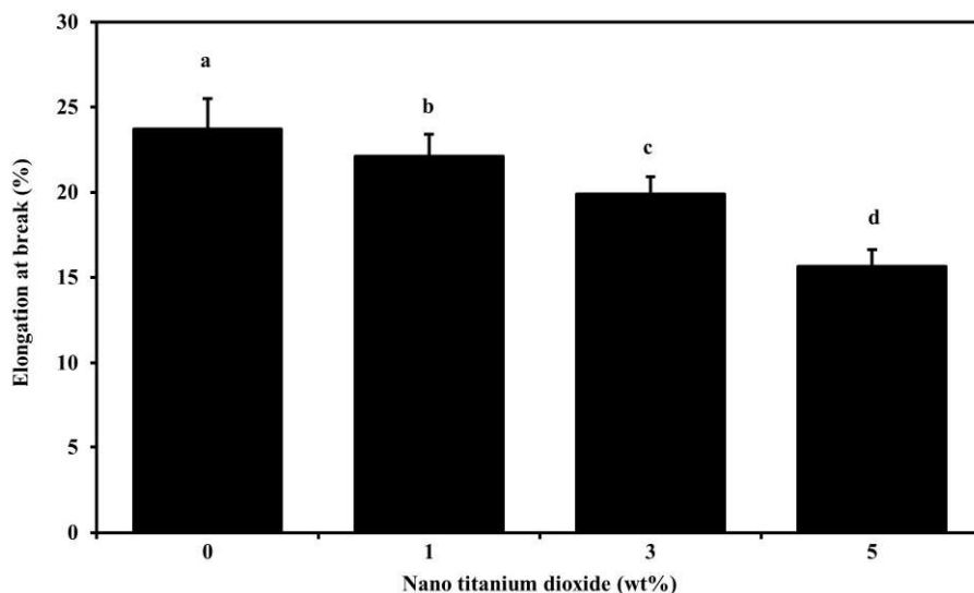
شکل (۲) نمودار درصد کشیدگی فیلم‌های نشاسته کاساوا و ژلاتین با غلظت‌های مختلف نانو دی اکسید تیتانیوم
