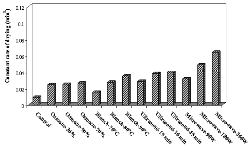
شکل (4) تغییرات آهنگ ثابت خشک شدن با استفاده از پیش تیمارهای مختلف در دمای 45 °C
