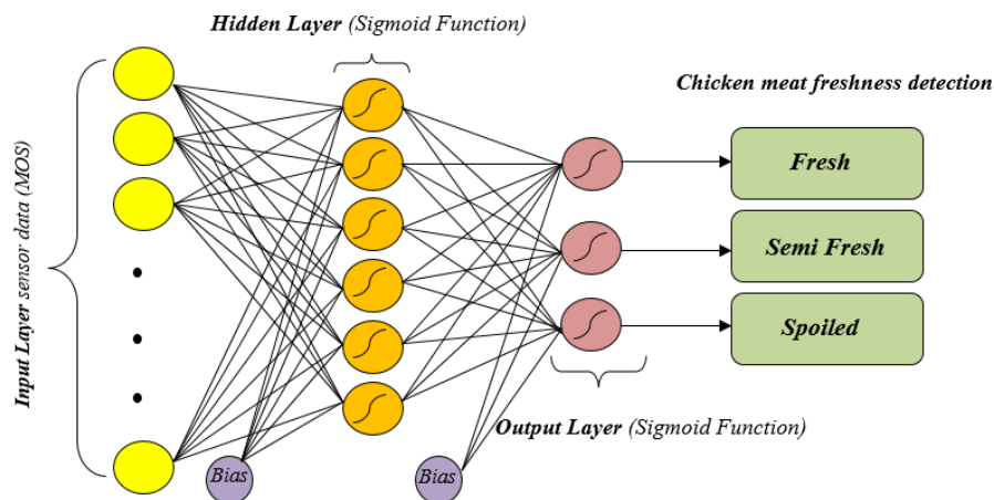
شکل (۷). بهترین ساختار شبکه برای تخمین و تشخیص تازگی گوشت مرغ Fig 7. The best topology of network for estimation and detection of chicken meat freshness
