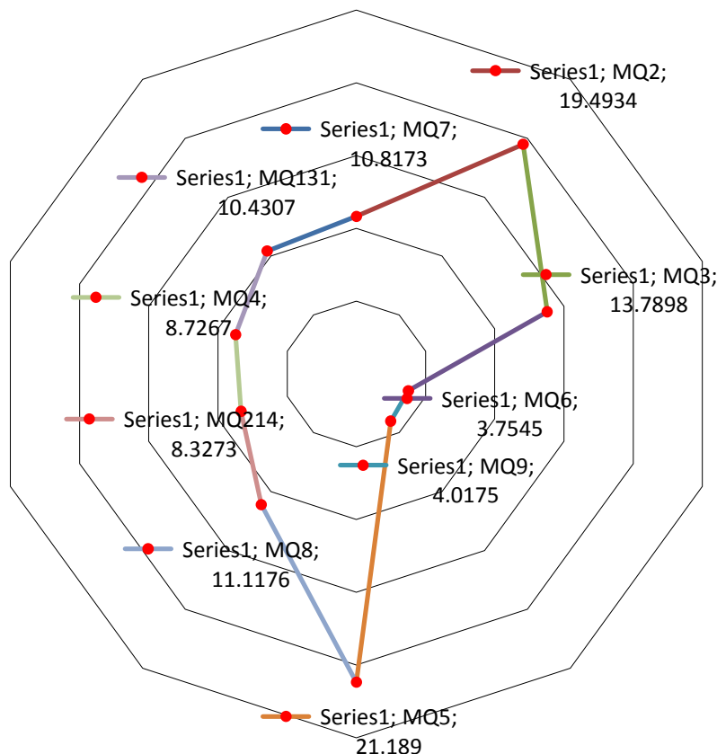
شکل (۵). نمودار رادار پاسخ حسگرها برای تشخیص تازگی گوشت مرغ Fig 5. Radar graph response of the sensors for estimation of chicken Freshness
