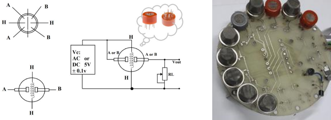
شکل (۳). مدار بندی و نحوه قرارگیری پایه‌های یکی از حسگرها Fig 3. Sensor circuitry and the method of placing the bases of a sensor.
