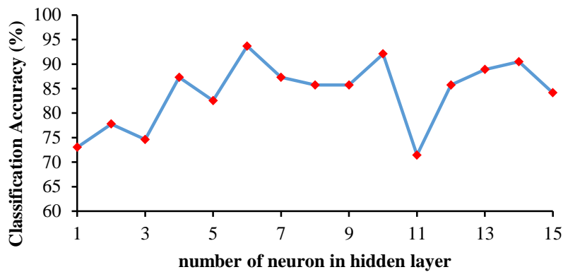
شکل (۶). مقادیر دقت کل طبقه‌بندی برای تعداد نرون متفاوت در لایه مخفی Fig 6. The classification accuracy for different number of neurons in the hidden layer
