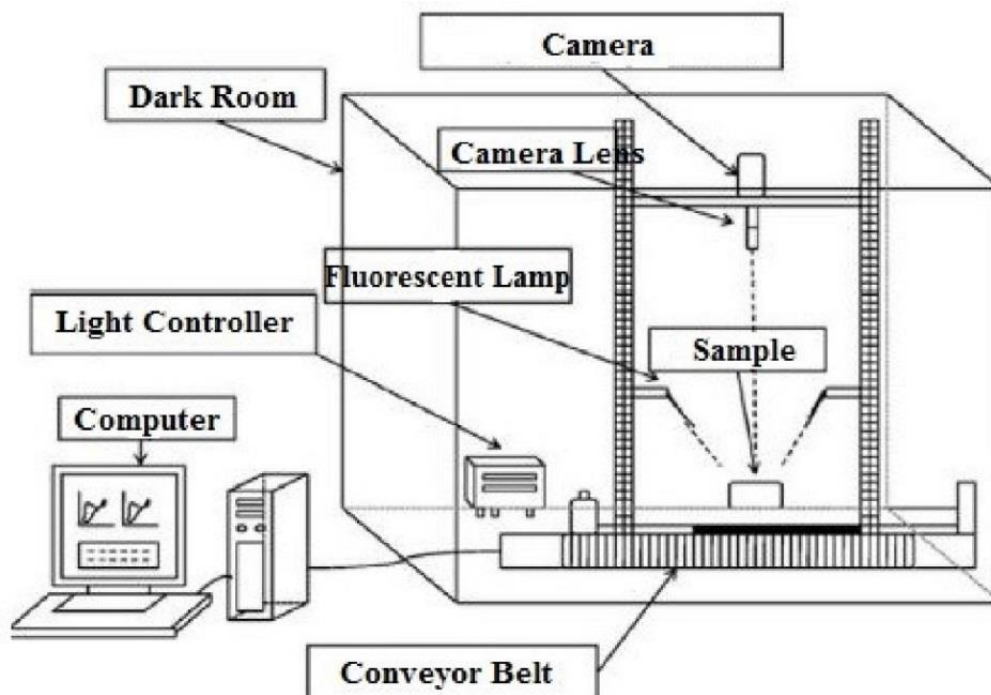
شکل (۱) تصویر شماتیک از سکوی تصویربرداری
